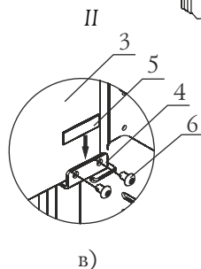
Рисунок 4. Установка дверцы на печь «Уренгой 2»
